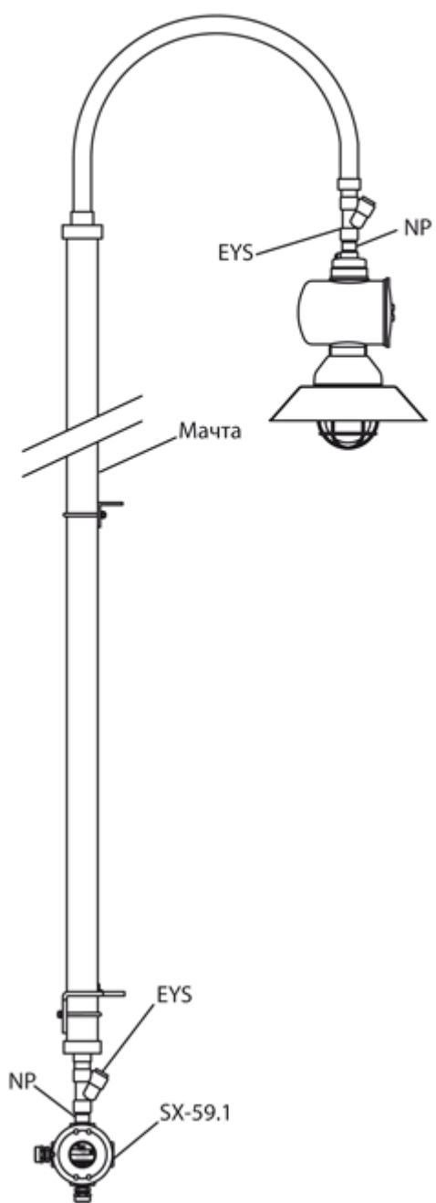
Крепление на мачте
